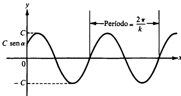
FIGURA 8.5 Movimiento armónico simple.
